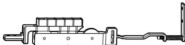
ROLL-LINE 120 réglable G-19797-25-0-6 Poids maxi par vantail 120 kg
