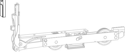
Chariot avant 6-30015-01-0-1
