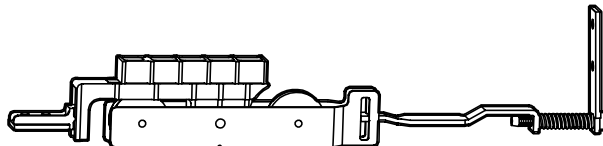
ROLL-LINE 120 regelbaar G-19797-25-0-6 Maximaal vleugelgewicht 120 kg
