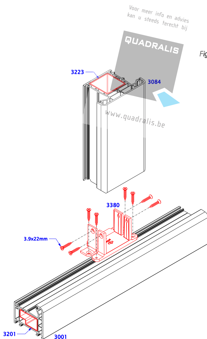
Fig. 1i add.4 : Afwerkingprofiel
