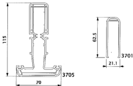
Fig. 1b add.4 : Koppelingprofielen
