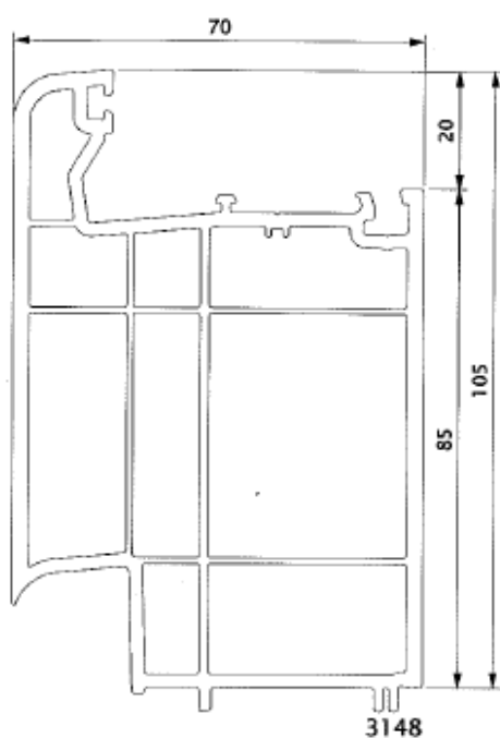
Fig. 1i add.4 : Afwerkingprofiel
