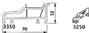
Fig. 1h add.4 : Dorpelprofiel
