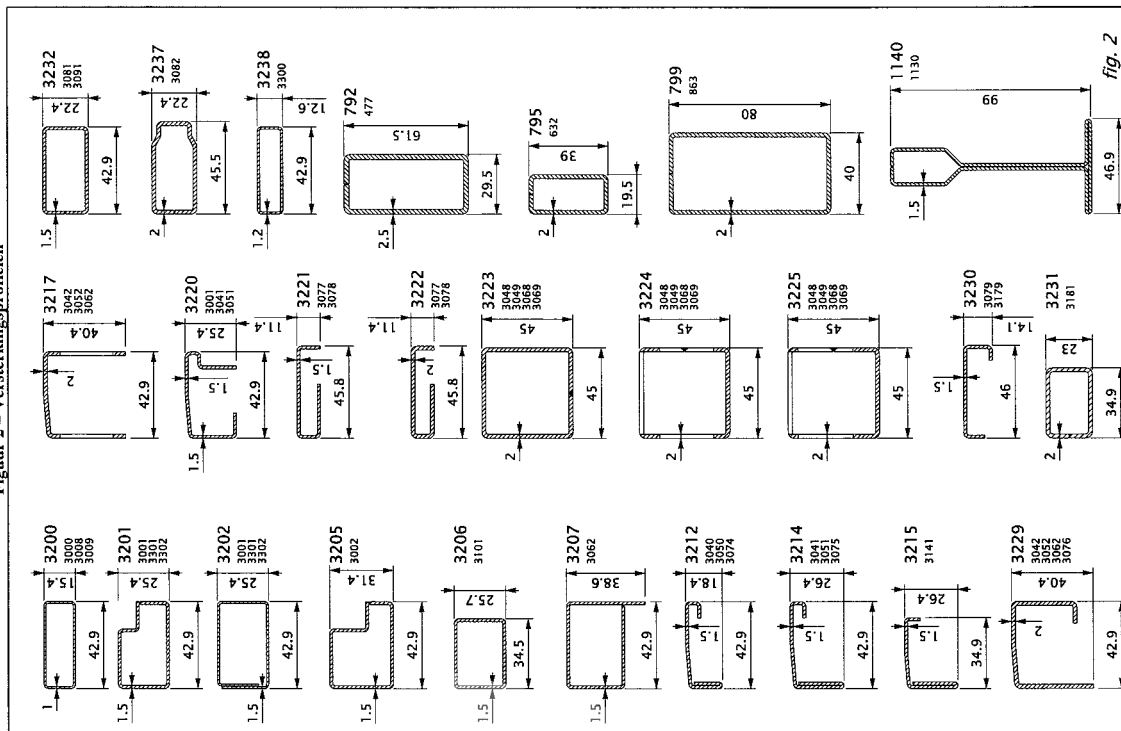
Figuur 2 – Versterkingsprofielen
