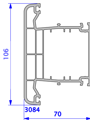
Fig. 1d add.4 : Middenstijl- of dwarsprofiel
