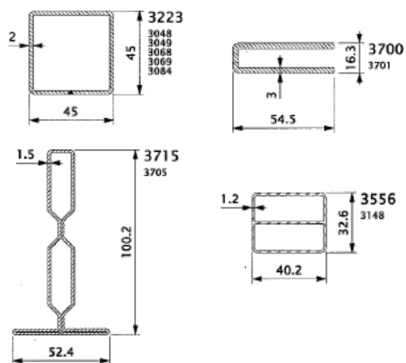
Fig. 2 add.4 : Versterkingprofielen
